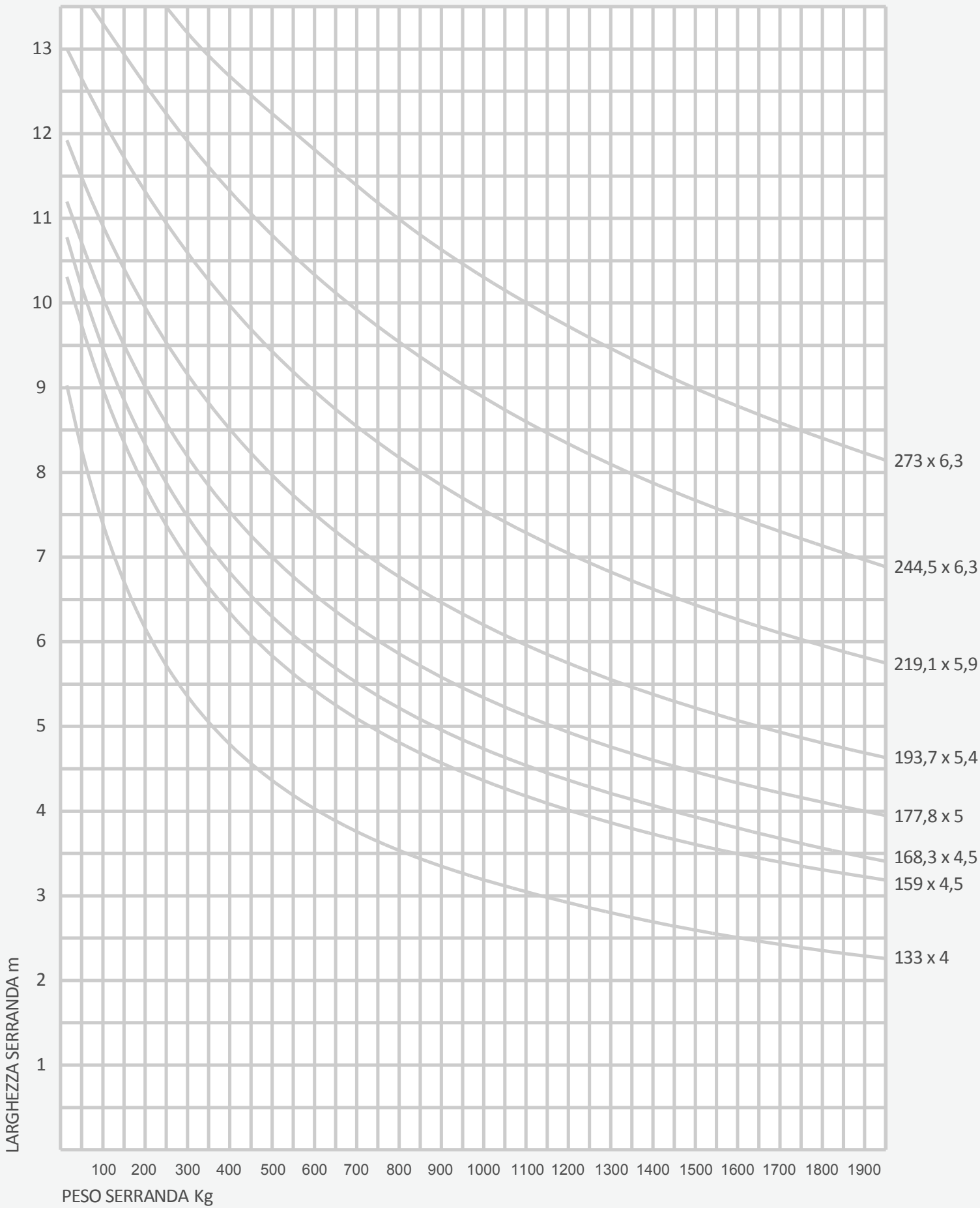
DIAGRAMMA PER LA CORRETTA SCELTA DEL DIAMETRO DEL TUBO
